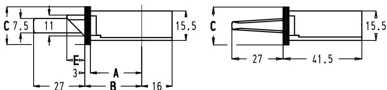
Vlakke voorplaat
